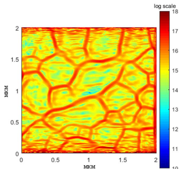
Рис. 5. Индекс изогнутости.
