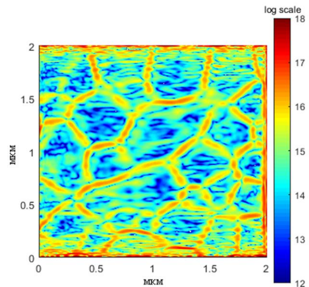
Рис. 4. Несферичность.
