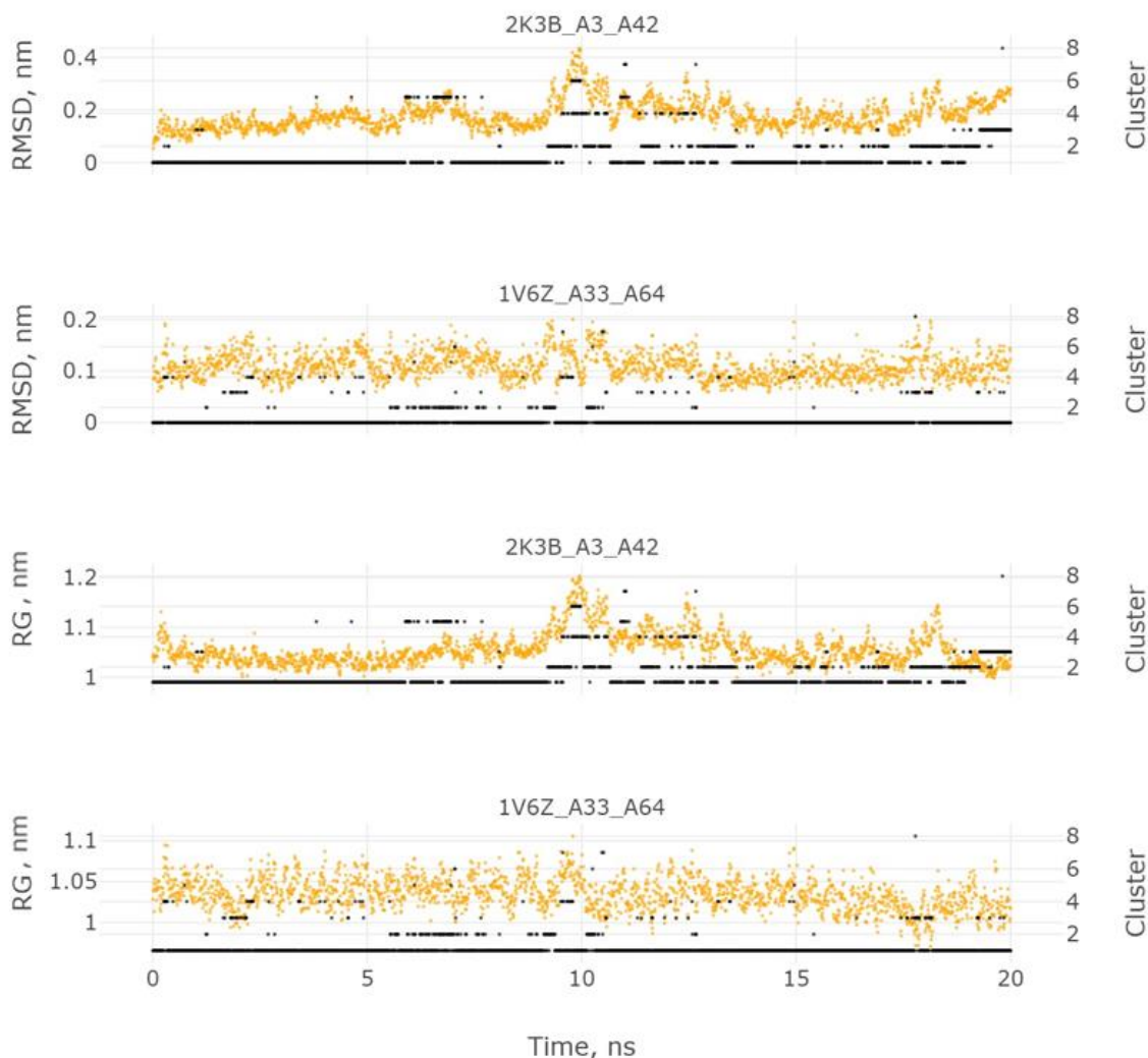
Рис. 2. Значения радиуса гирации (Rg), RMSD (желтые точки) и населенности мажорного кластера (черные точки) в ходе «короткого» эксперимента молекулярной динамики для \beta -углов PDBID2K3B цепь A (C \alpha : 3–42) и PDBID 1V6Z цепь A (C \alpha : 33–64). Над рисунками даны названия структур, ось OX – продолжительность эксперимента, 20 нс. Ось OY – значения RMSD и Rg, нм.
